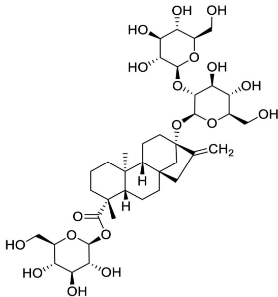
Stevioside (5)
