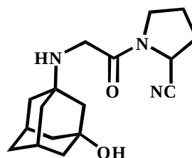
Vildagliptin, Mol. Wt.: 305.42
