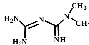
Metformin, Mol. Wt.: 129.16
