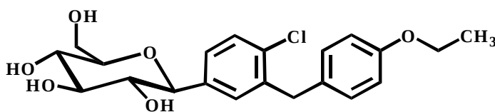
Dapagliflozin, Mol. Wt.: 408.90
