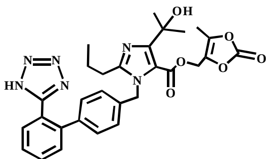
Olmesartan medoxomil, Mol. Wt.: 558.59
